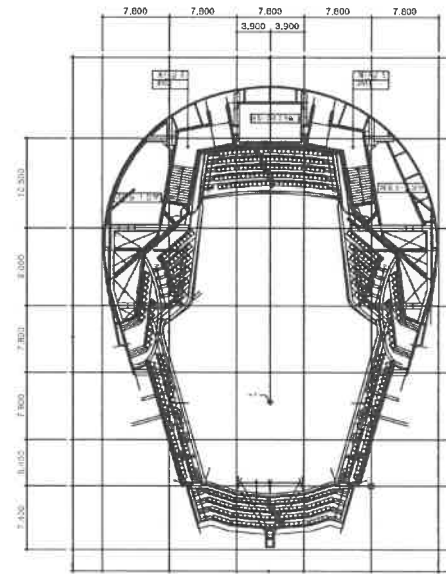
지상 중2층 확대평면도(EL+16.26)
